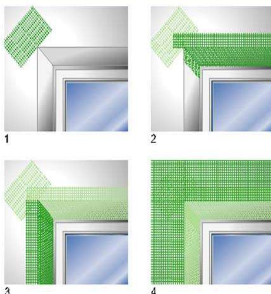
Obr. 8: Dodatečné vyztužení rohů oken a dveří
