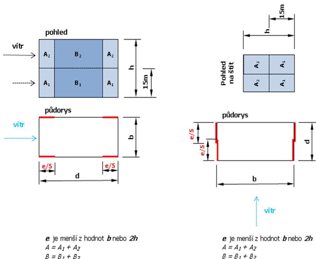
Obr. 7: Grafické znázornění jednotlivých parametrů pro stanovení okrajové a vnitřní oblasti plochy
